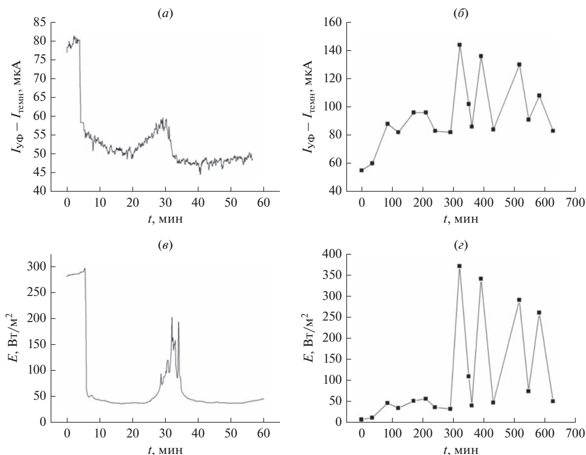
Рис. 6. Изменение электропроводности от времени облучения сенсора солнечным излучением: а) в течение 1 ч, б) в течение 10 ч; изменение энергетической освещенности в диапазоне УФ-А спектра солнечного света: в) в течение 1 ч, г) в течение 10 ч.
