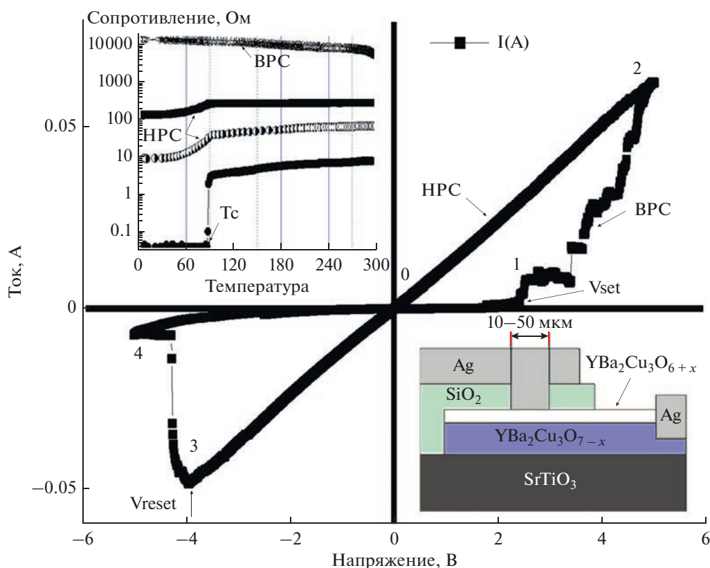
Рис. 1. Пример ВАХ гетероструктур планарного типа \text{Ag}/\text{YBa}_2\text{Cu}_3\text{O}_{6+\delta}/\text{YBa}_2\text{Cu}_3\text{O}_{7-\delta}/\text{STO} , выполненных методом фотолитографии. Развертка напряжения была по направлениям ветвей: 0–1–2–0–3–4–0. В правом нижнем углу показана схема структуры, сформированной литографией. В левом верхнем углу показана температурная зависимость сопротивления метастабильных фаз и резистивный переход пленки YBCO в сверхпроводящее состояние при T_c .
